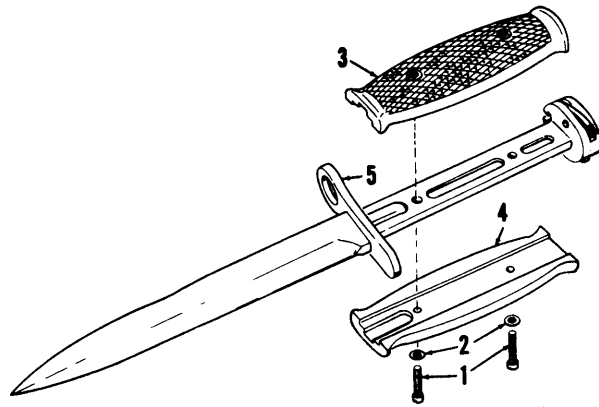
BAYONET - KNIFE M4
